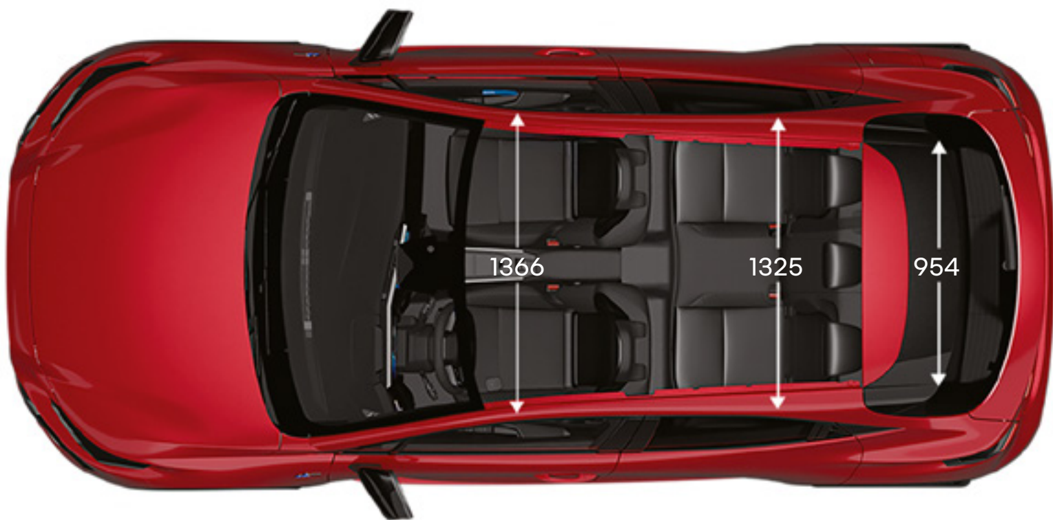
izmēri (mm)
